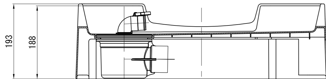
断面A-A
