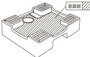
●本体底面部 図1
