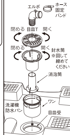
●トラップ組立図 図3
