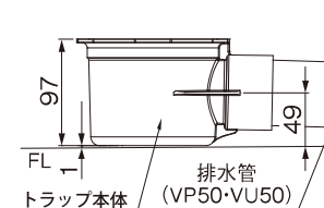
●トラップの施工 図4
