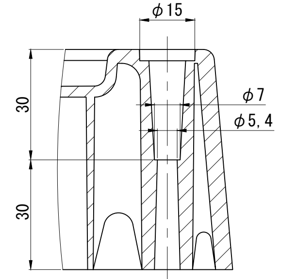
ビス部詳細 S=1:1
