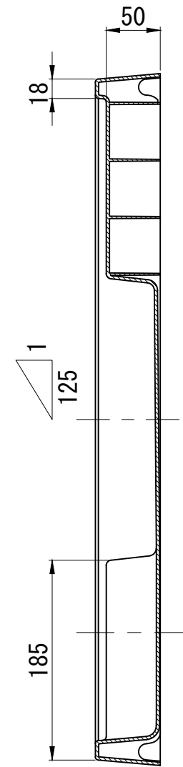
断面 A-A
