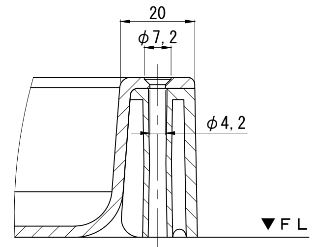
ビス部詳細 S=1:1
