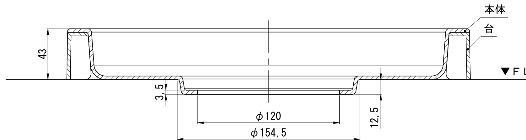
断面A-A
