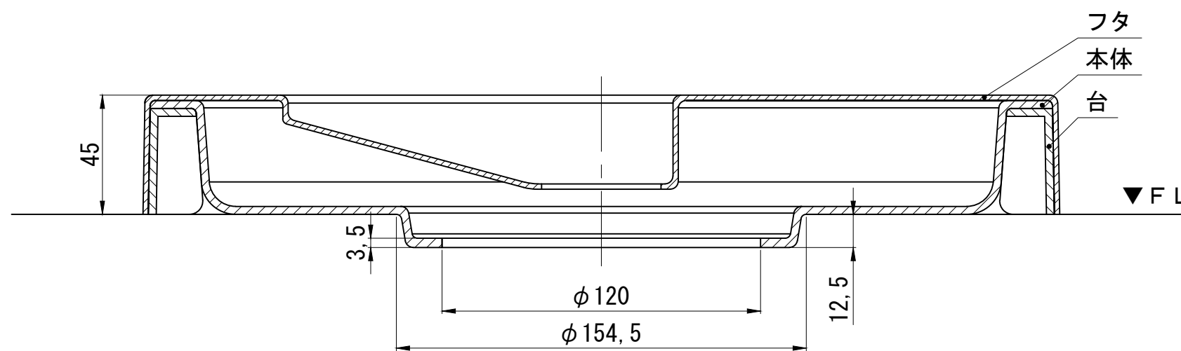
断面A-A
